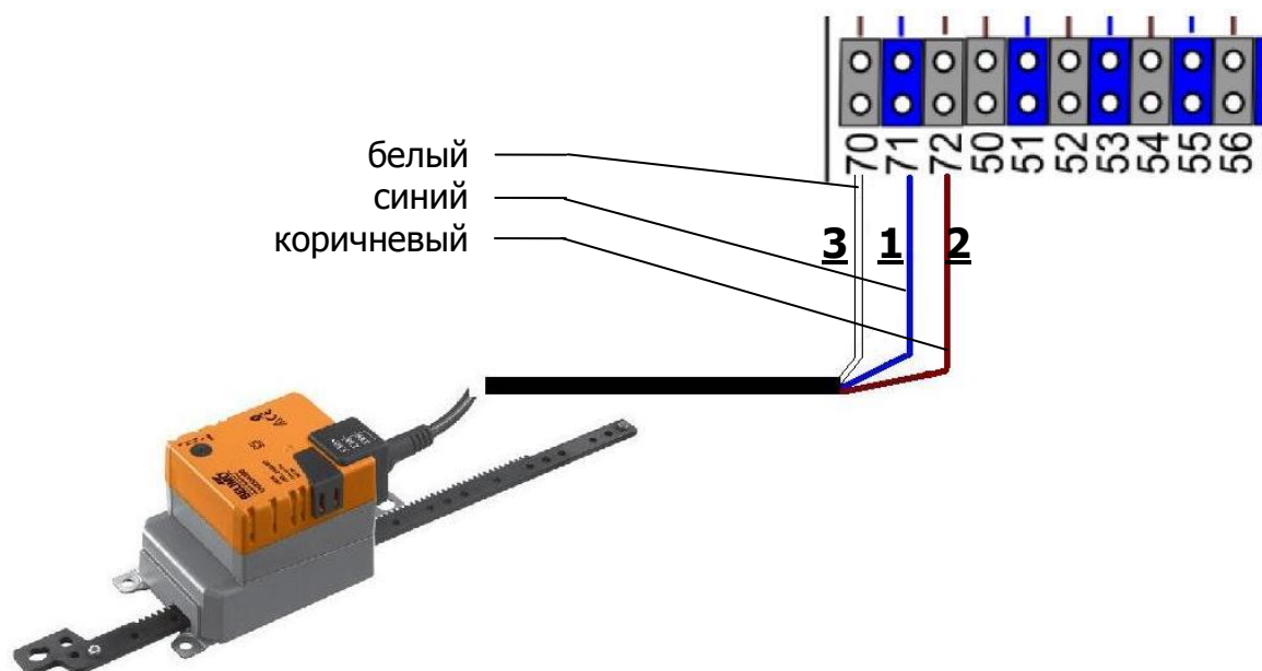
Рис.2.7. Схема подключения серводвигателя Belimo к шкафу управления.
