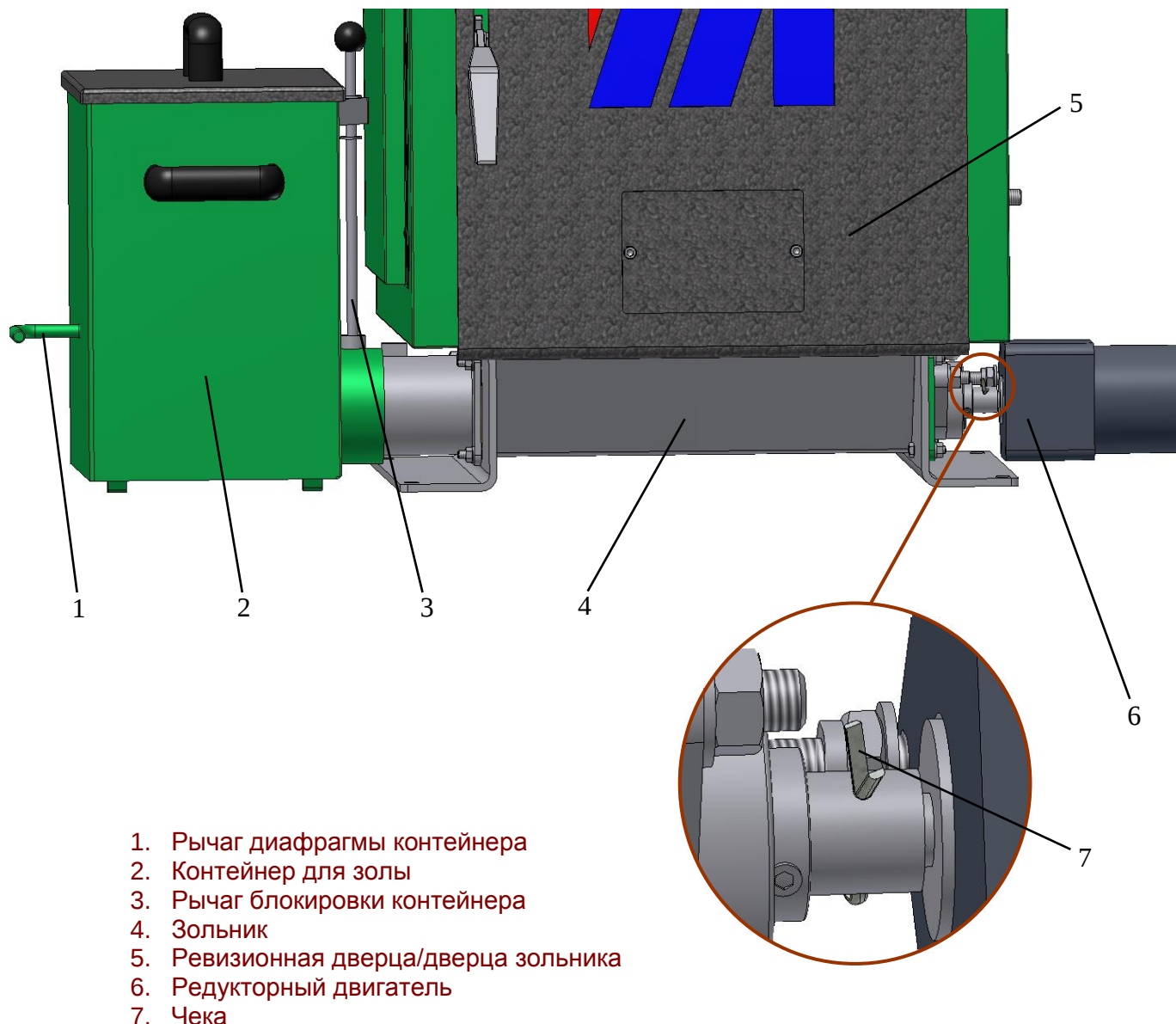
Рис. 4. Внешний вид теплообменника Vento Eko с системой удаления золы.
