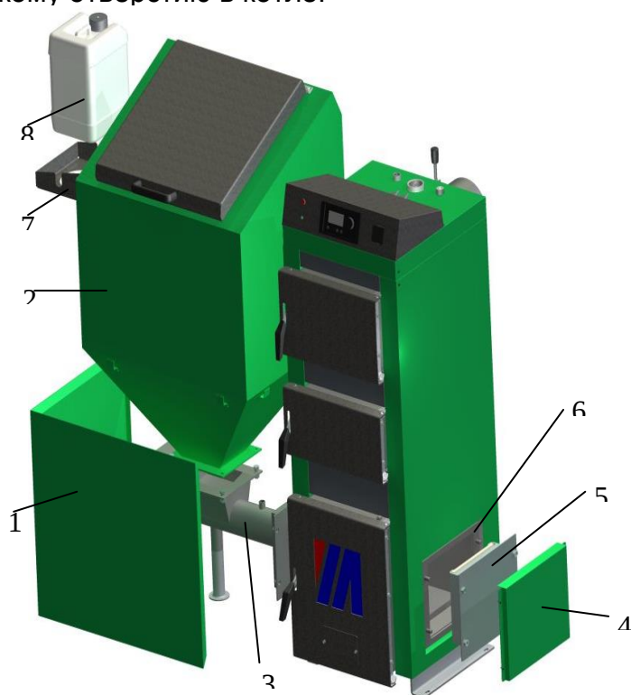
Рис. 10. Демонтаж бункера.
