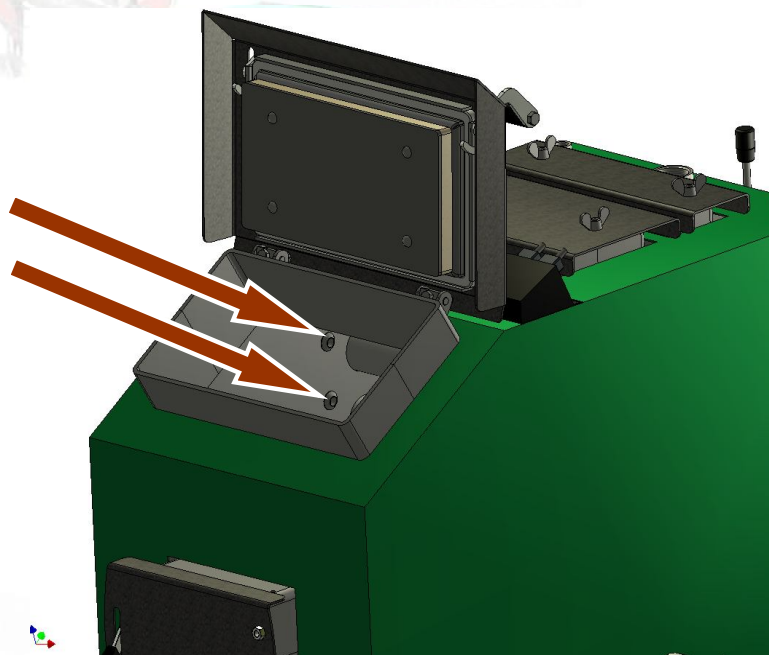
Рис.14. Чистка сопел со стороны камеры горения
