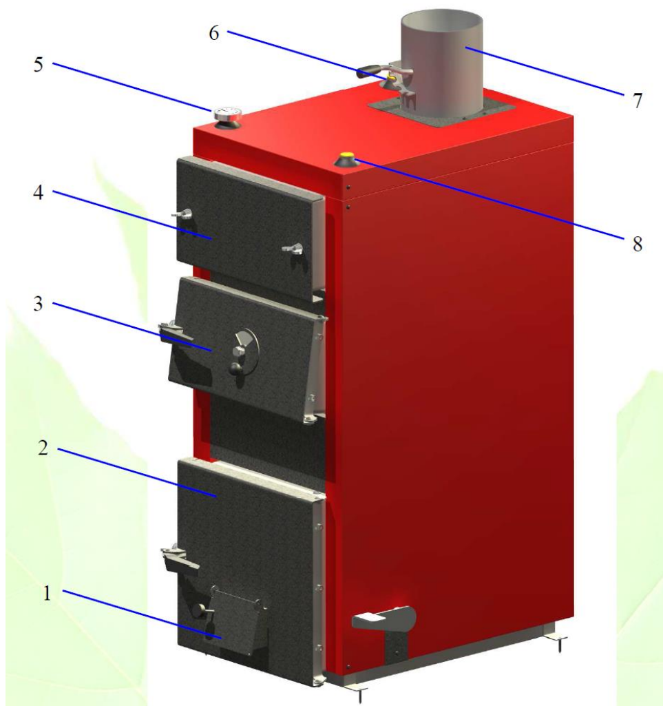
Rys.1. Котел тип MODERATOR – описание главных частей.
