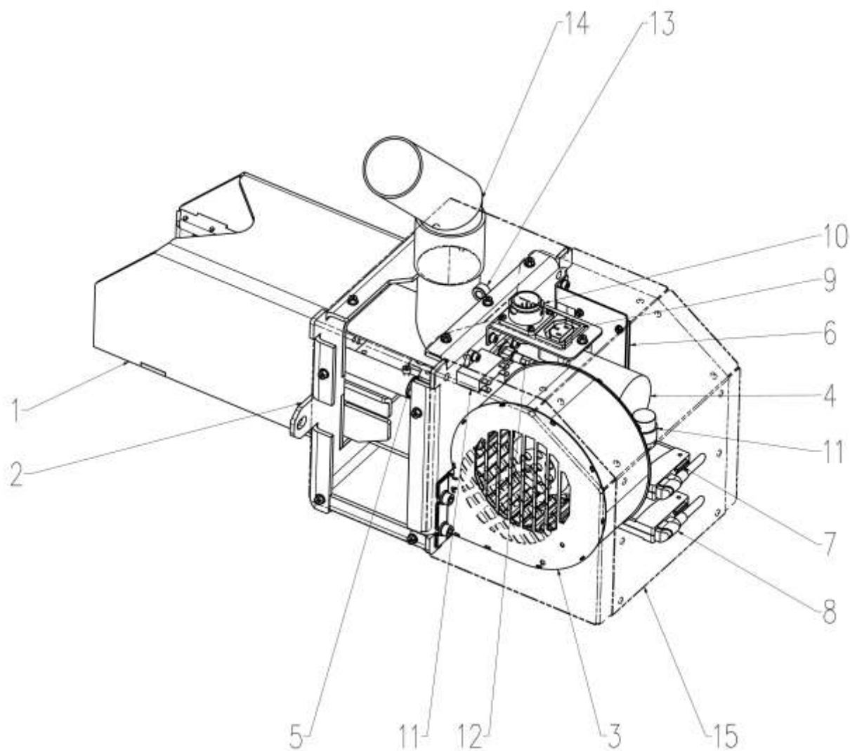
Рис.1.2. Строение горелки Moderator 30
