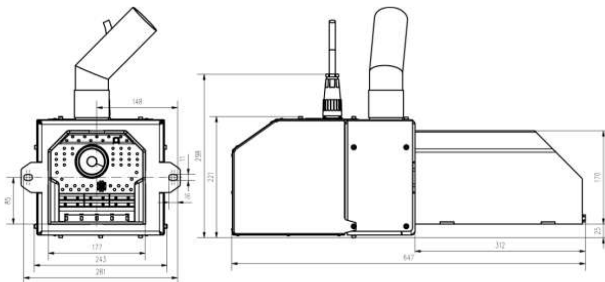
Рис.1.3. Основные размеры горелки 60 kW
